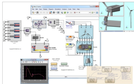
Abb. 1: Modell für die virtuelle Inbetriebnahme eines Steuerungssystems einer WEA (©MATLAB)
